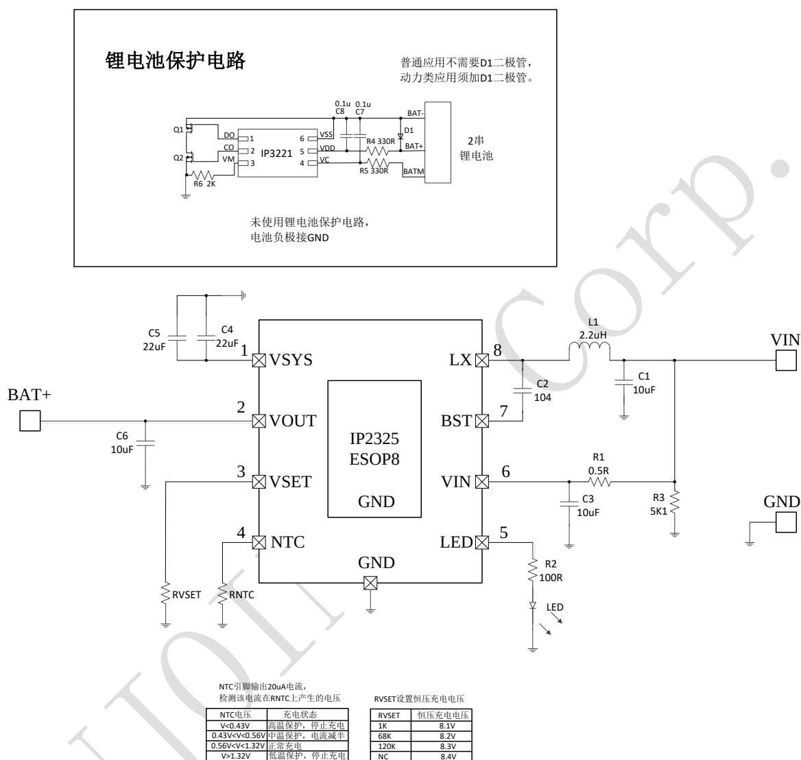
图 6 典型应用原理图
