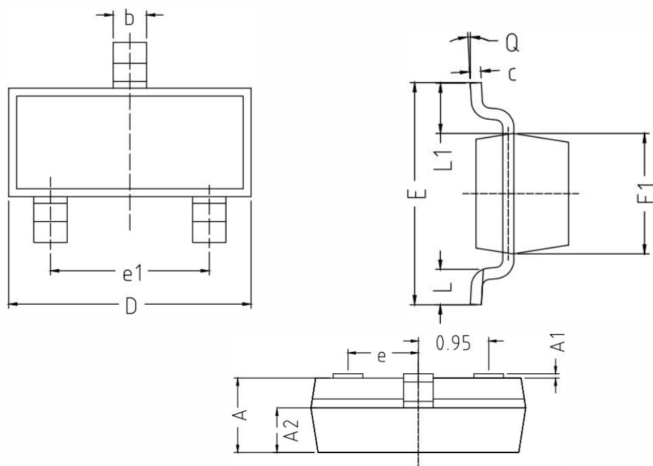
SOT-23 PKG
