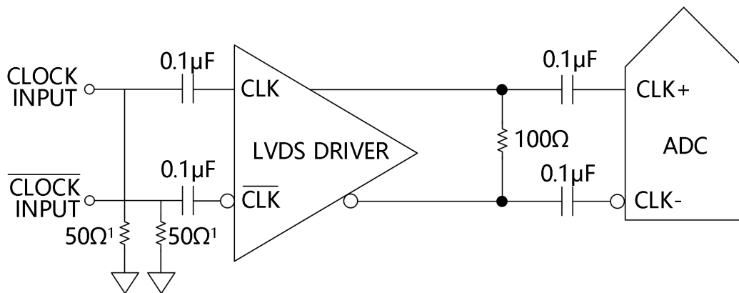
图 14. 时钟 LVDS 信号激励方案
