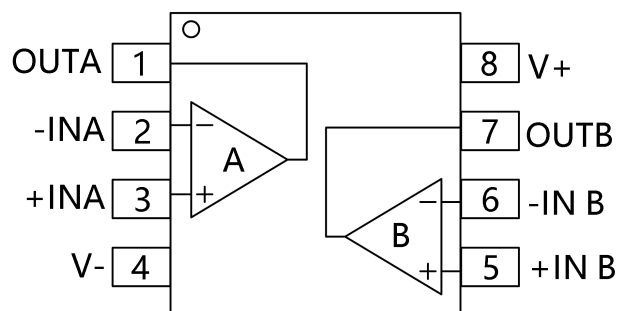
SOIC-8(SOP8),MSOP-8
