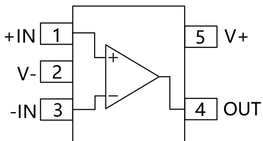
SOT23-5
