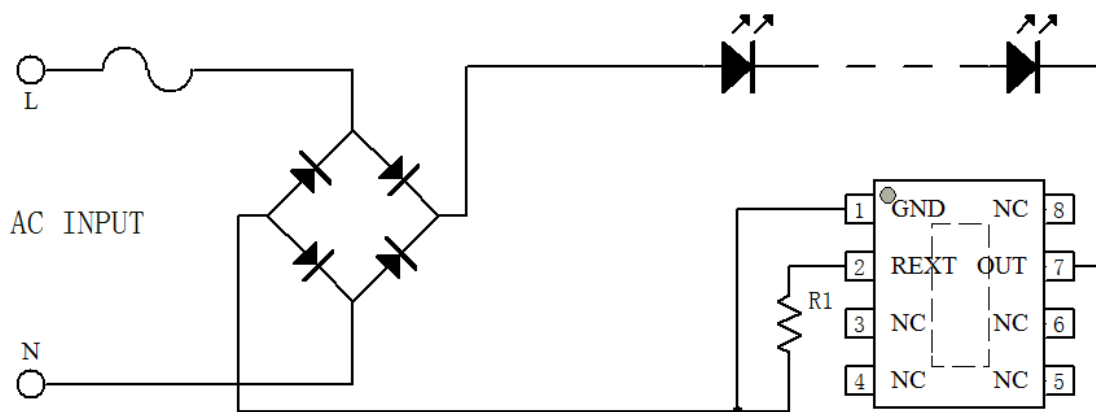
ZM3535BAH典型应用原理图
